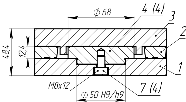
A-A (1 : 2)
