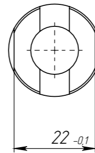
H (1 : 1)
