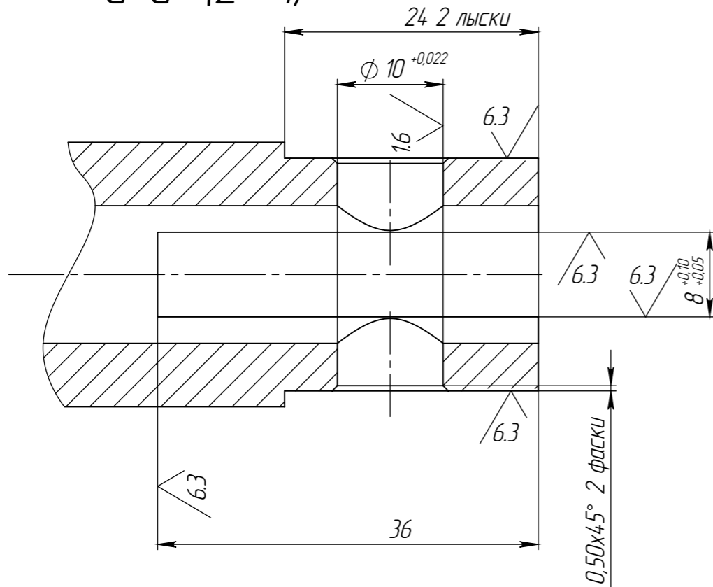
G-G (2 : 1)
