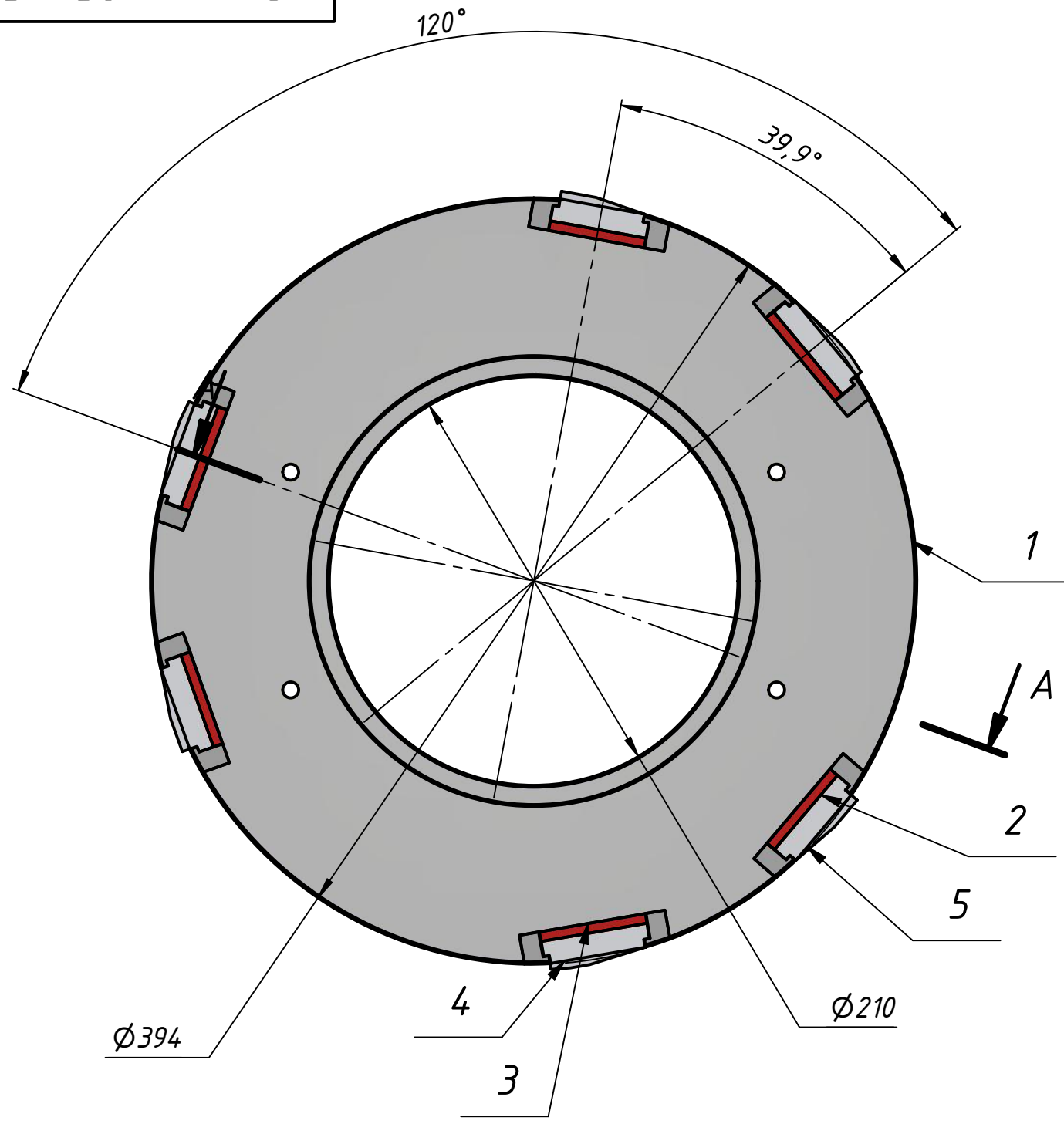
A-A (1:3)
