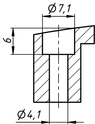
A-A (2:1)
